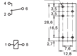
Anschlußbelegung/interne Verdrahtung/(Ansicht von unten)
