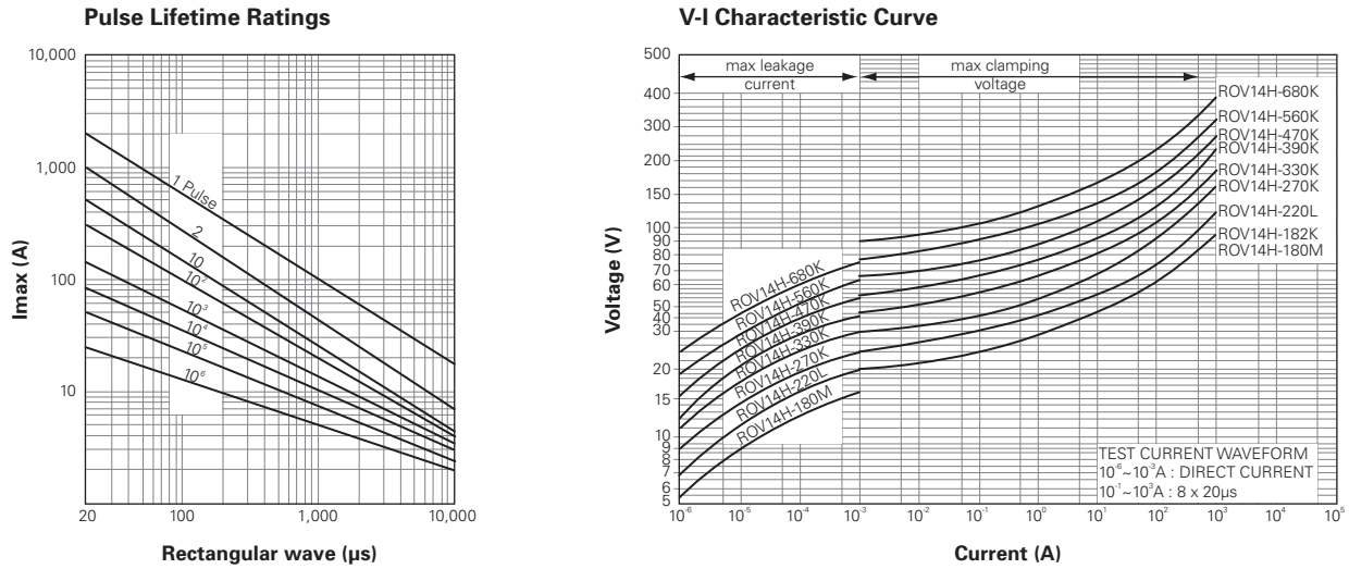
Figure V24 - ROV14H820K-ROV14H511K
