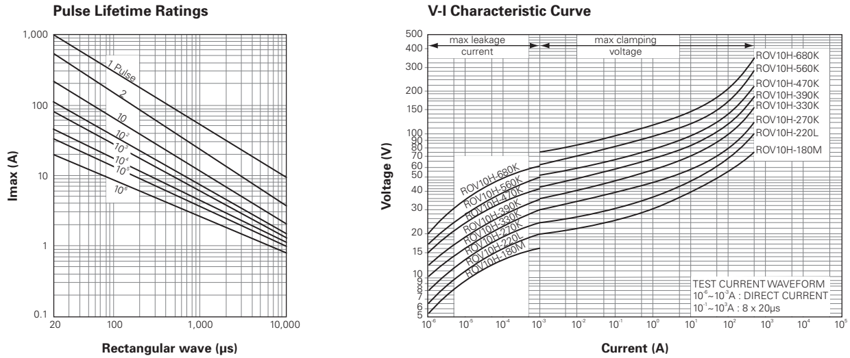
Figure V21 - ROV10H820K-ROV10H511K
