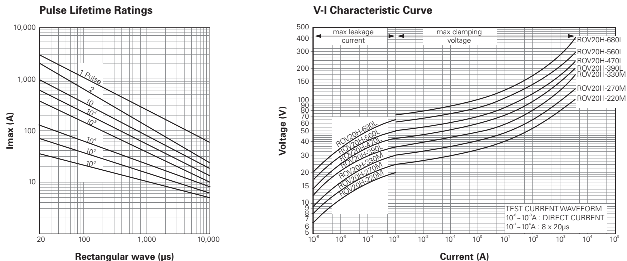
Figure V27 - ROV20H101K-ROV20H511K
