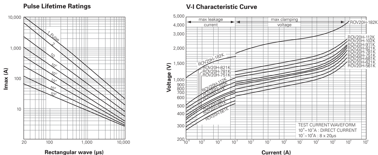
Figure V28 - ROV20H561K-ROV20H182K
