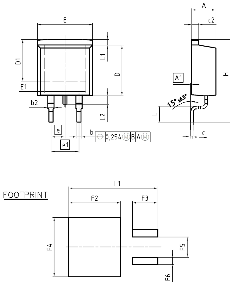
PG-TO-263-3-2
