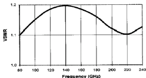
VSWR
