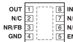
DRB PACKAGE 3mmx 3mm SON (TOP VIEW)
