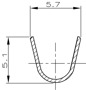
SEZIONE C-C (SECTION C-C)
