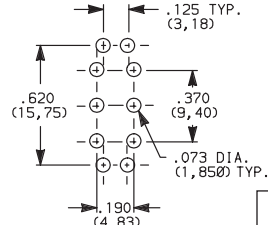
7201J1__BE2 DPDT
