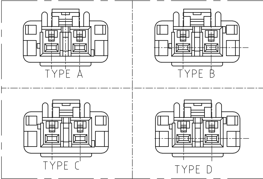
キーイングタイプ THE TYPE OF KEYING
