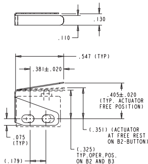
A1-101-02 Shown
