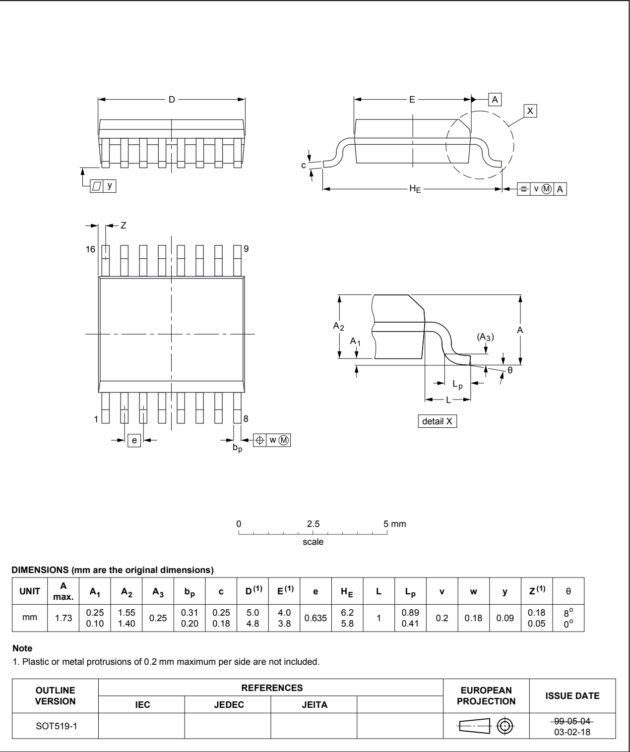
Fig. 20. Package outline SOT519-1 (SSOP16)
