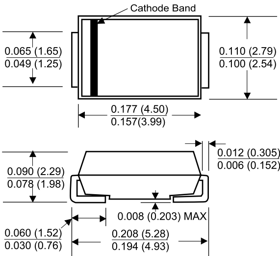
DO-214AC (SMA)
