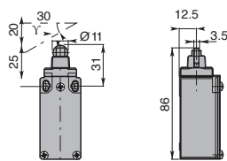
Pole Plunger
