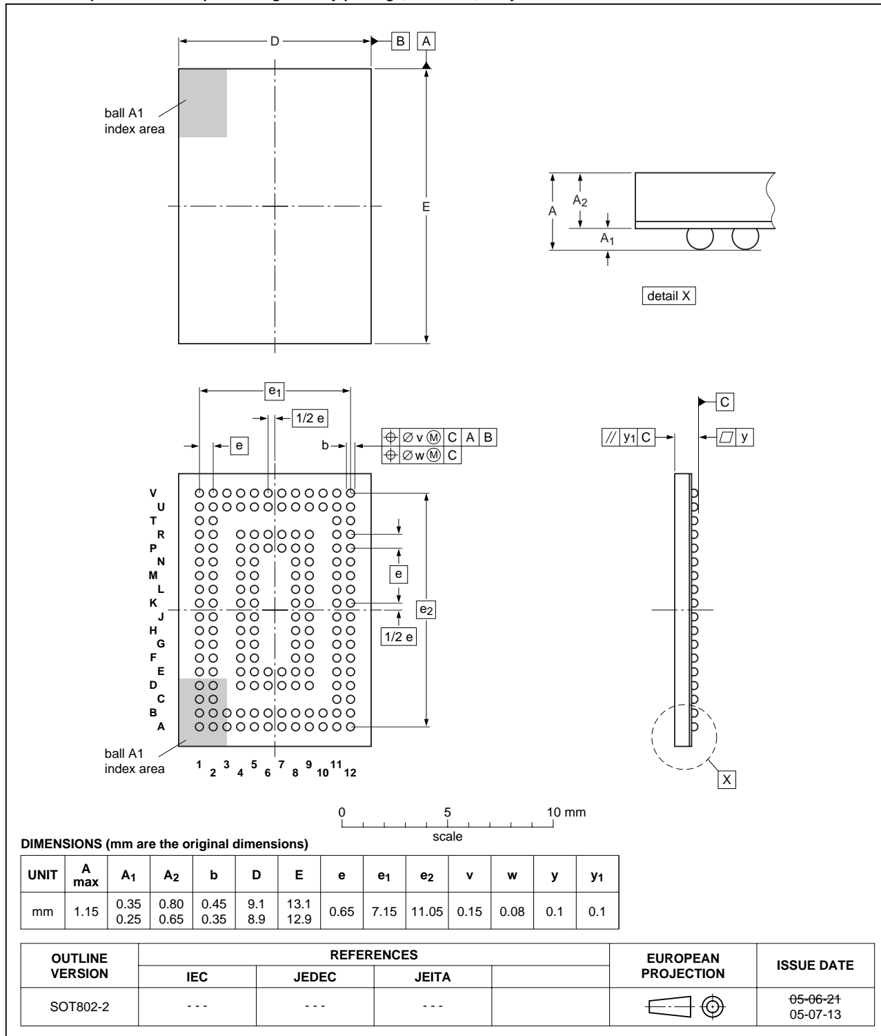
SOT802-2
