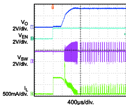
EN start up I_o = 20mA
