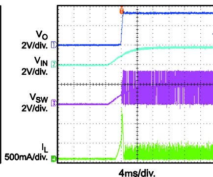
Vin Start up I_o = 20mA
