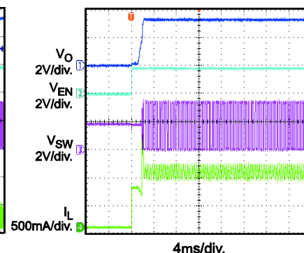
EN start up I_o = 500mA
