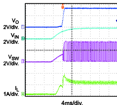
Vin Start up I_o = 500mA
