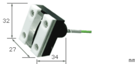
Model MG-11K-TS1-ANP
