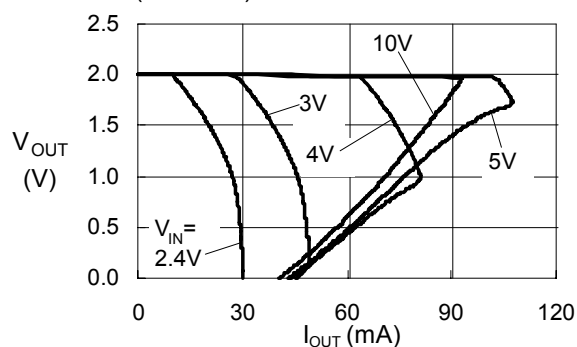
S-817A20A(Ta=25°C)
