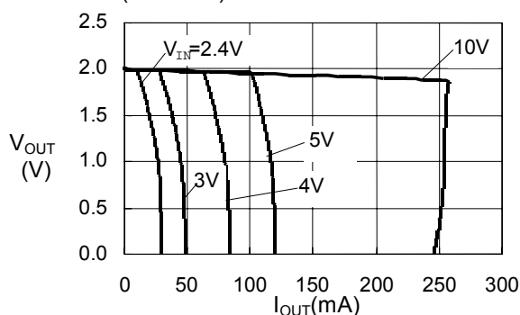
S-817B20A(Ta=25°C)
