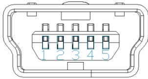
Figure 13: Mini USB Connector
