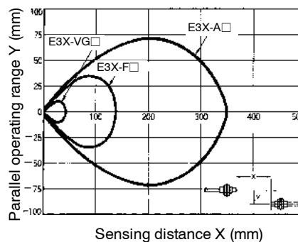
E32-TC200A with E3X-A, E3X-F, and E3X-VG amplifiers
