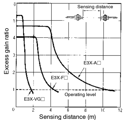
E32-T17L with E3X-A, E3X-F and E3X-VG amplifiers
