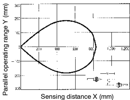
E32-TC200 with E3X-NV amplifier
