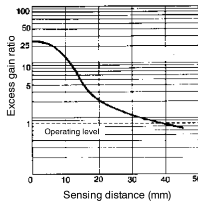
E32-DC200 with E3X-DA amplifier
