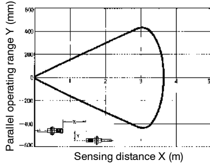
E32-T11L with E3X-NVG amplifier
