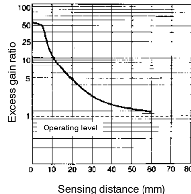
E32-D73 with E3X-A11 amplifier
