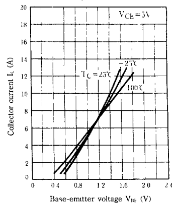
I_C - V_{BE}
