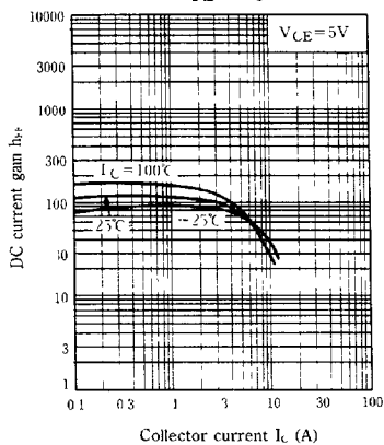
h_{FE} - I_C
