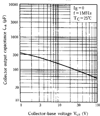
C_{ob} - V_{CB}
