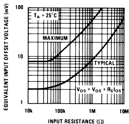
Offset Error
