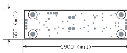
Module Dimensions
