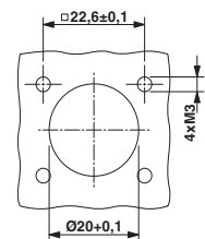
Einbaumaße: SF-EP1N8AAK00
