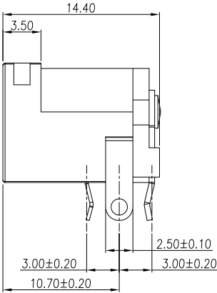
SEC: A-A
