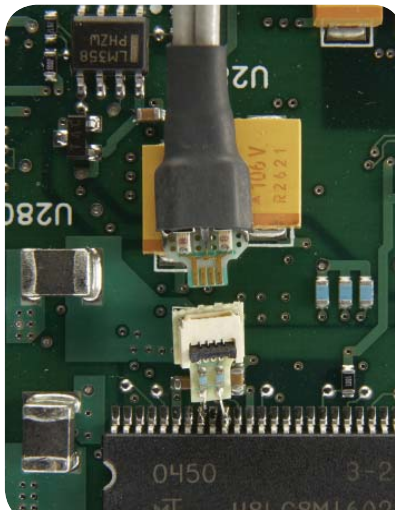
InfiniiMax ZIF tip soldered on board
