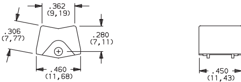
J50 ROCKER
