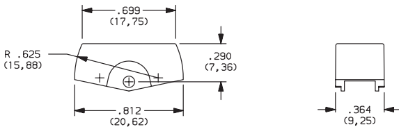
J8 ROCKER
