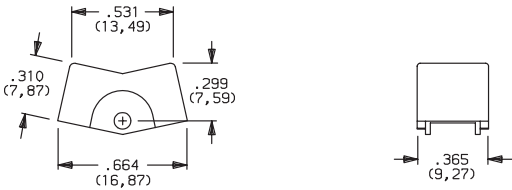
J1 ROCKER
