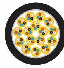
Schnittzeichnung
