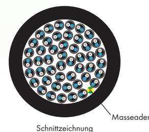
Schnittzeichnung
