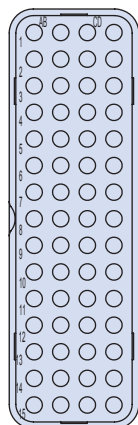
Insert 01 60 #22
