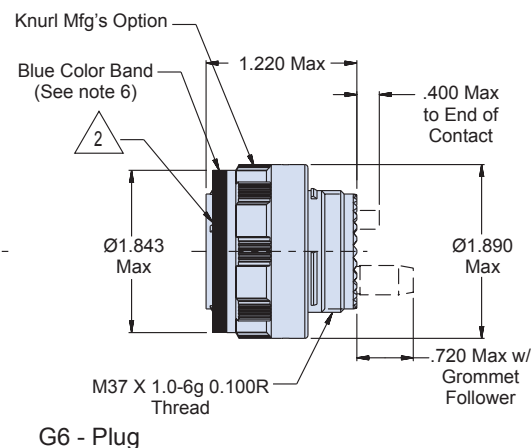
G6 - Plug
