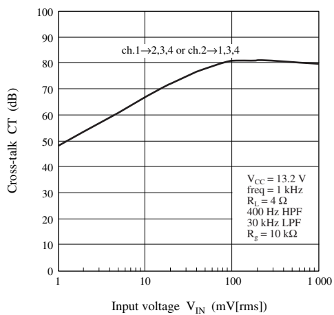
CT — V_{IN}
