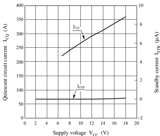
I_{CQ} , I_{STB} — V_{CC}
