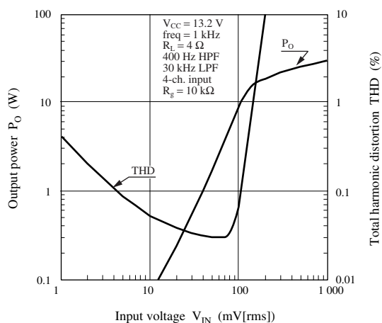
P_O , THD — V_{IN}
