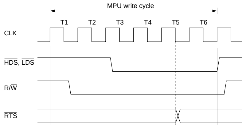
(d) CPU Mode 2, MPU Write Cycle
