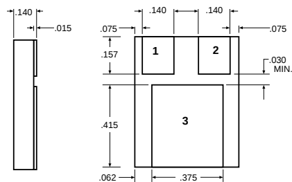
OM1324NMM
