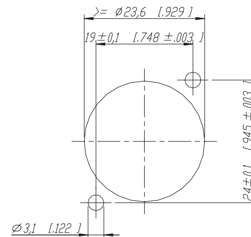
Frontplattensusschnitt (Rückseite) Panel cut out (rear side)
