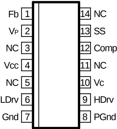
14-Pin SOIC NB (S)
