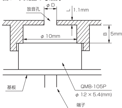
図6 共鳴器の寸法例
