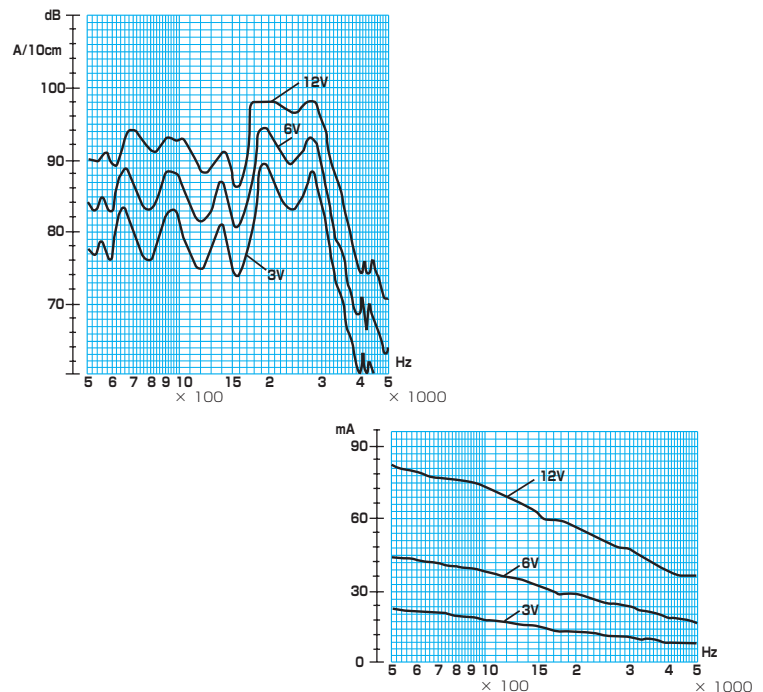
図3 電圧変化による周波数特性変化例
