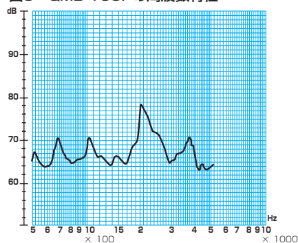
図5 QMB-105Pの周波数特性
