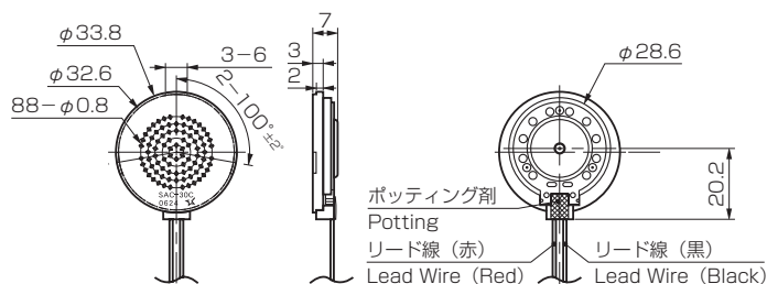
外径寸法図 [ size : φ33.8×7mm ]
