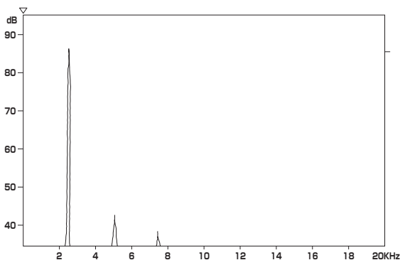
図4 圧電ブザー FFT分析
