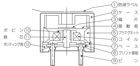
図1 マグネチックサウンダ構造図
