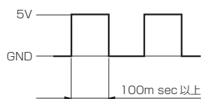
図5 応答時間例
