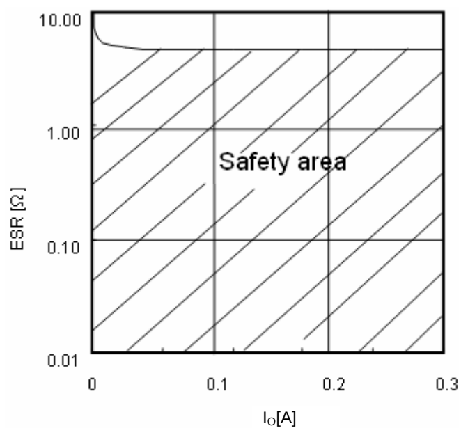
Fig.19 ESR condenser
