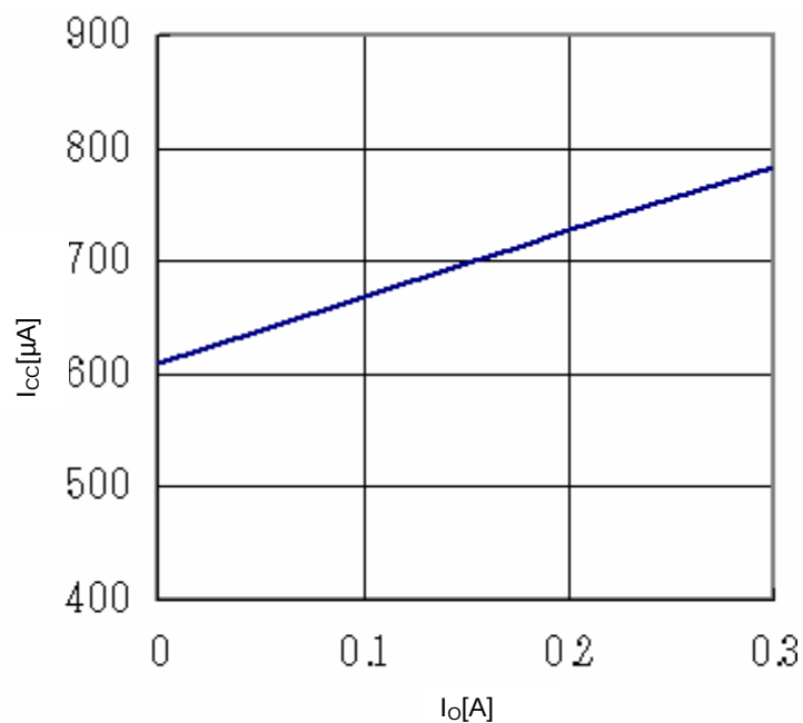
Fig.20 I_o - I_{cc}
