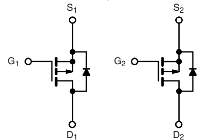
P-Channel MOSFET
