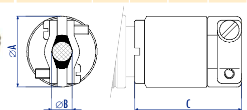
Serre-câble allongé, nickelé, à visser
