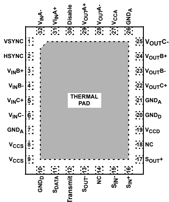
ISL59311 (32 LD QFN)
