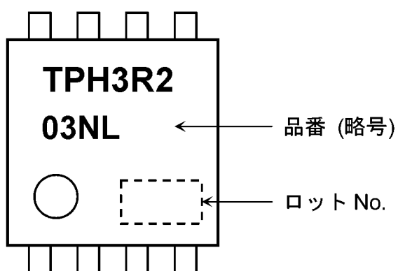
図 7.1 現品表示
