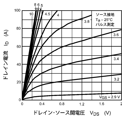
図 8.2 I_D - V_{DS}
