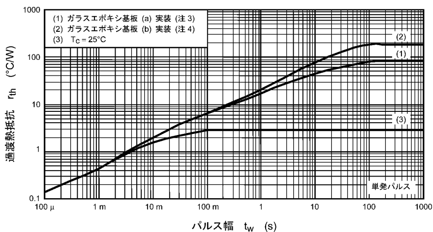
図 8.13 r_{th} - t_w (最大值 (保証値))
