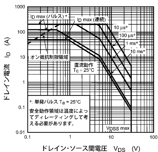
図 8.14 安全動作領域 (最大值 (保証値))
