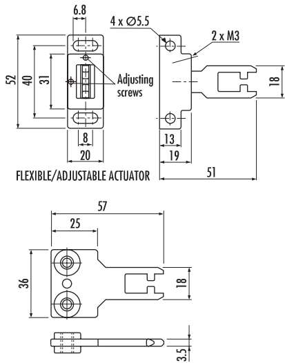
FLAT ACTUATOR
