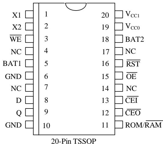
20-Pin TSSOP
