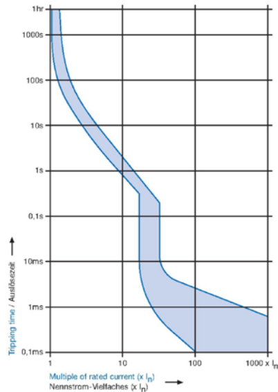
Tripping characteristic DH Auslösekennlinie DH
