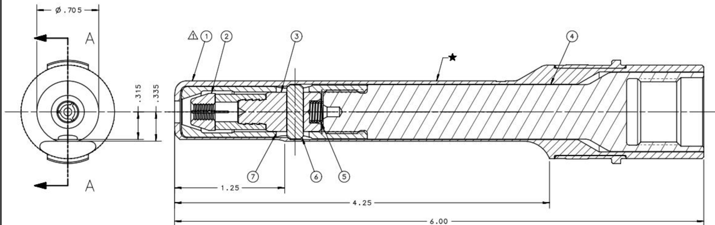
SECTION A-A
