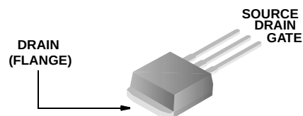
JEDEC TO-262ABA
