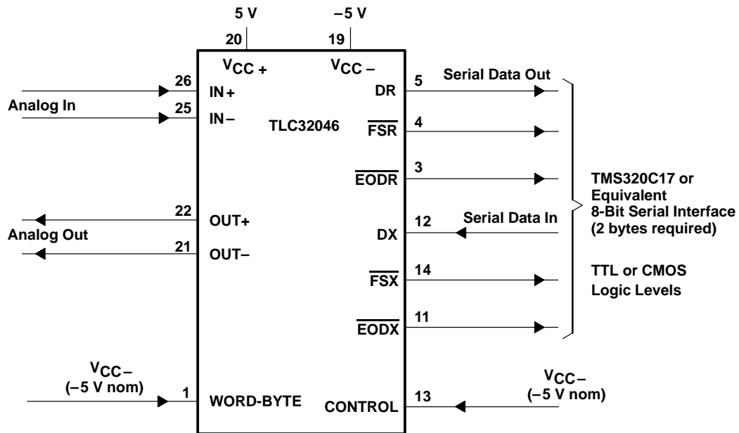
Figure 1-3. Byte Mode
