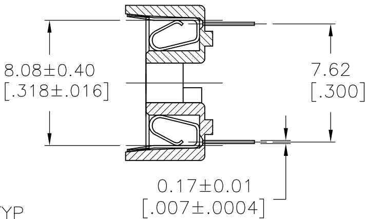
SECTION D-D
