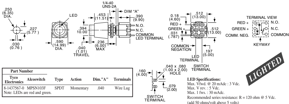
SPDT/DPDT
