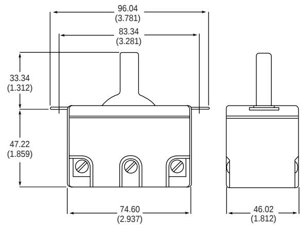
7811K2 — 2PDT
