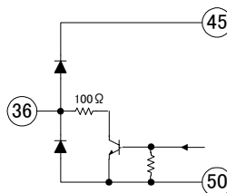
36; DAC 2
