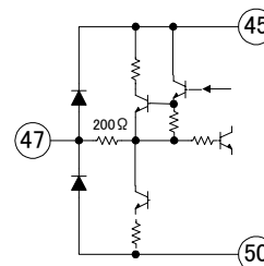
47; V OUT
