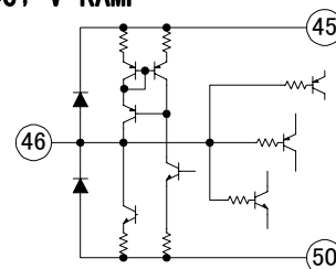
46; V RAMP
