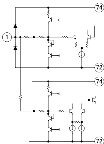
1: IF AGC
