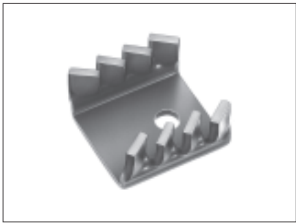
FK 228 SA L 1 30 K/W
