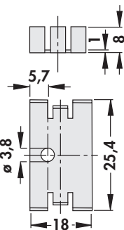
FK 209 SA 32 25 K/W
