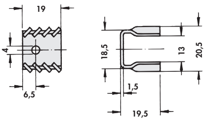
FK 230 SA L 1 21 K/W
