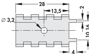
FK 235 L 2 ... SOT 32
