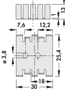
FK 214 SA CB 15 K/W
