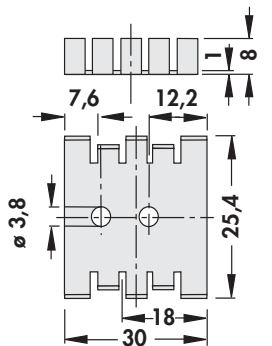
FK 210 SA CB 18 K/W
