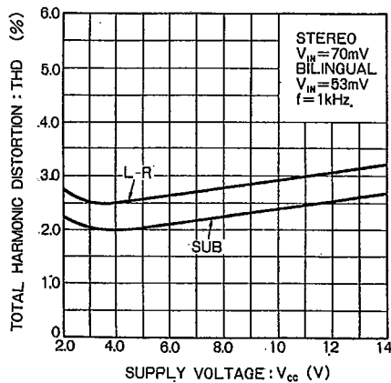
Fig. 11 全高調波歪—電源電圧
